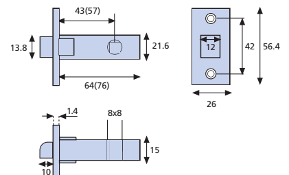
Tubular Latch
