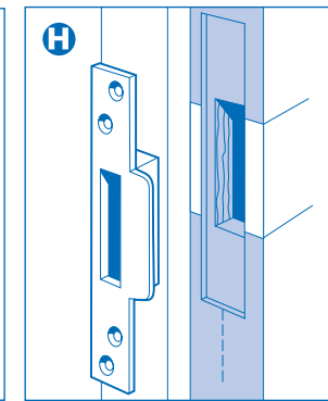
Fit Box Striker
